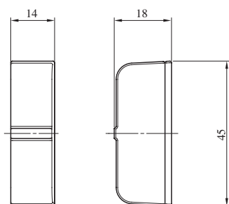
ドア開閉検知用マグネット (注4)
