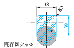
追加切欠参考図 (青線) (既存LA錠の場合)
