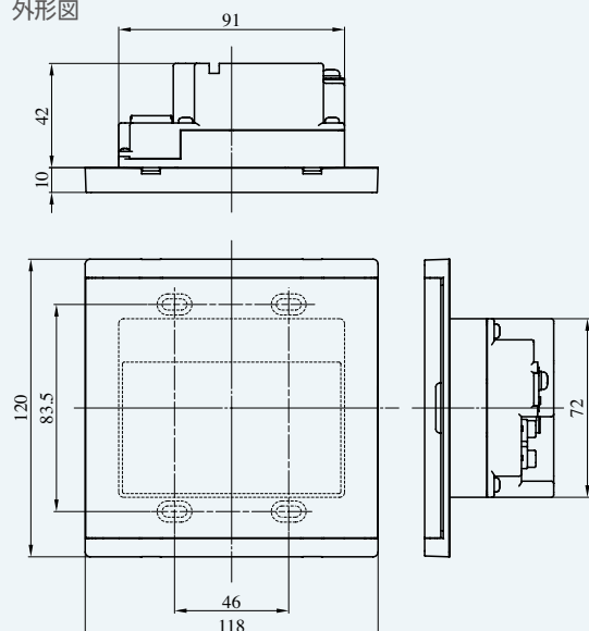
外形図
