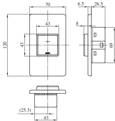
壁面取付の場合
