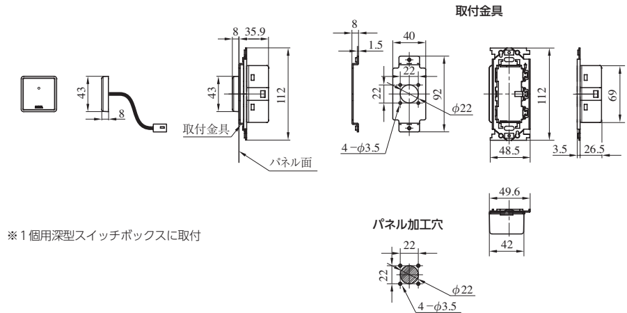
集合玄関機のパネル取付の場合
