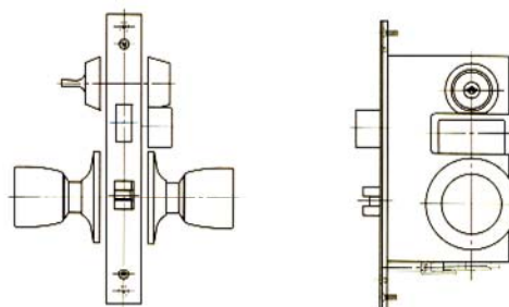
●非常開装置側のシリンダーリング寸法(単位mm)
