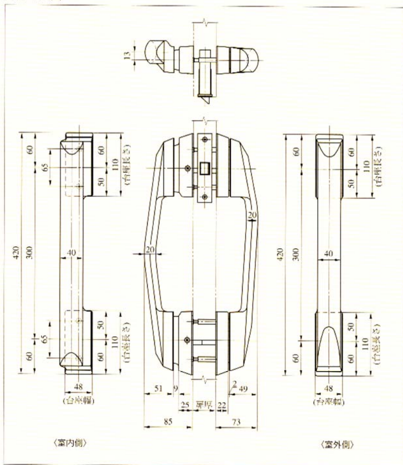
外形寸法図
