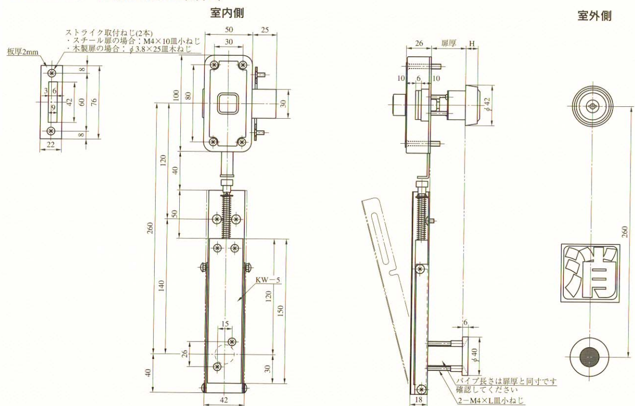
扉切欠図(室内側)
