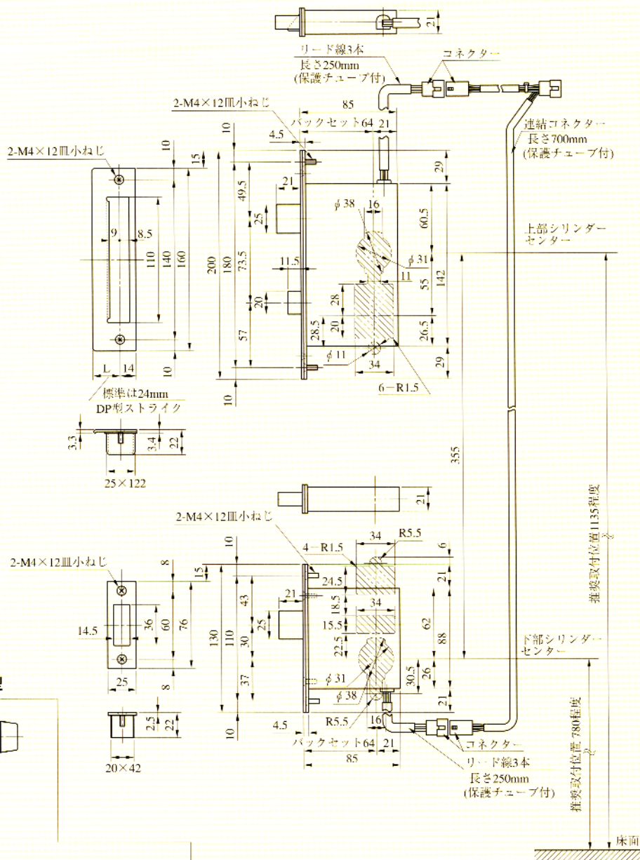
【外形寸法図】 PRPGZ704DW-1型
