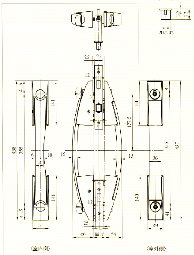
【外形寸法図】 PRPGZ704DW-1型
