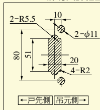
POM811 扉切欠詳細図
