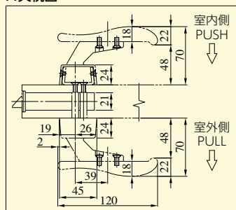
A矢視図
