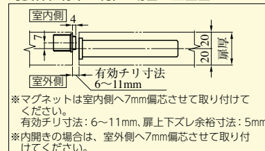
対震枠仕様 (G1付) の場合の上面図
