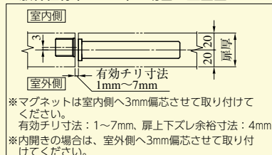
一般枠仕様 (G1なし) の場合の上面図
