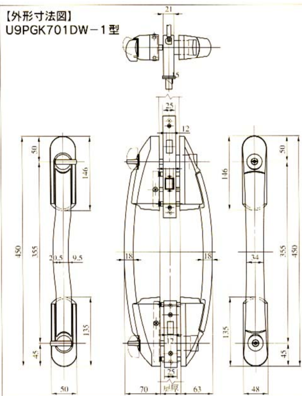
【外形寸法図】 U9PGK702DW-1型
