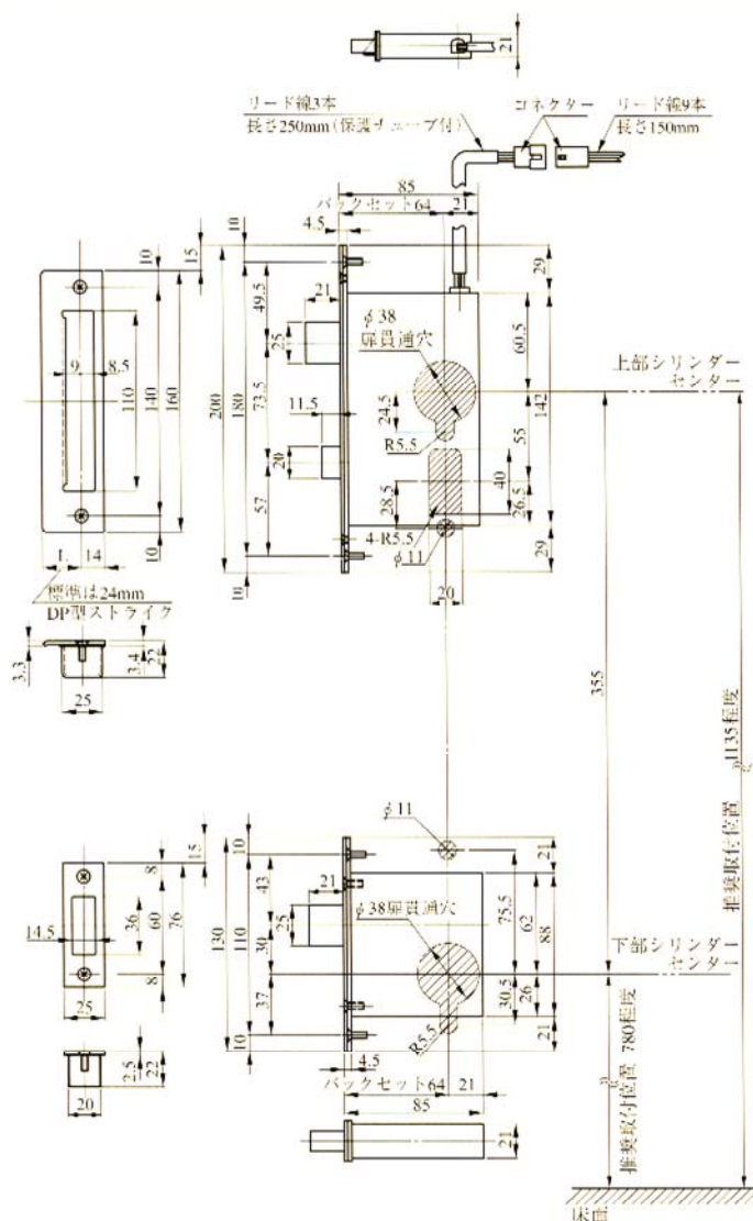
【外形寸法図】 U9PGK701DW-1型
