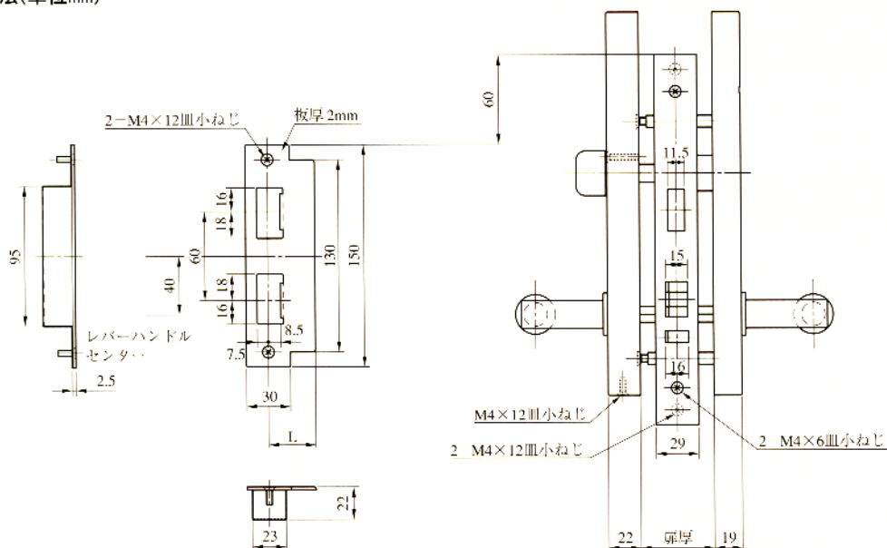
扉切欠図
