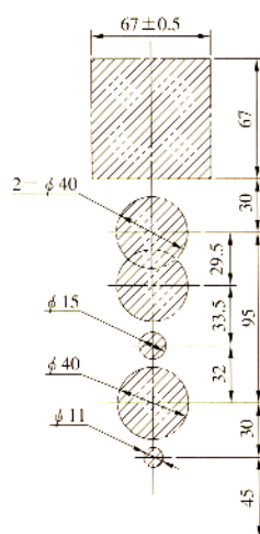
扉切欠図
