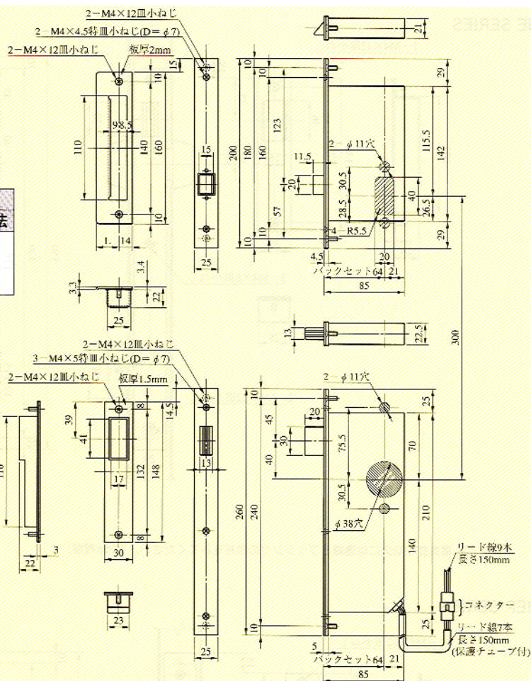
【外形寸法図】 U9ALPG702S-1 型
