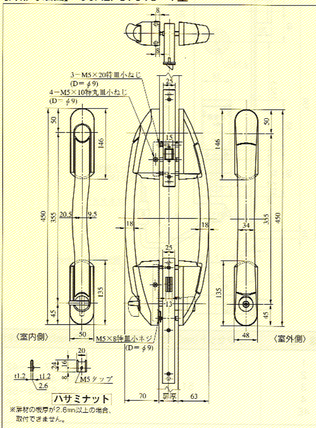
【外形寸法図】 U9ALPG701S-1型
