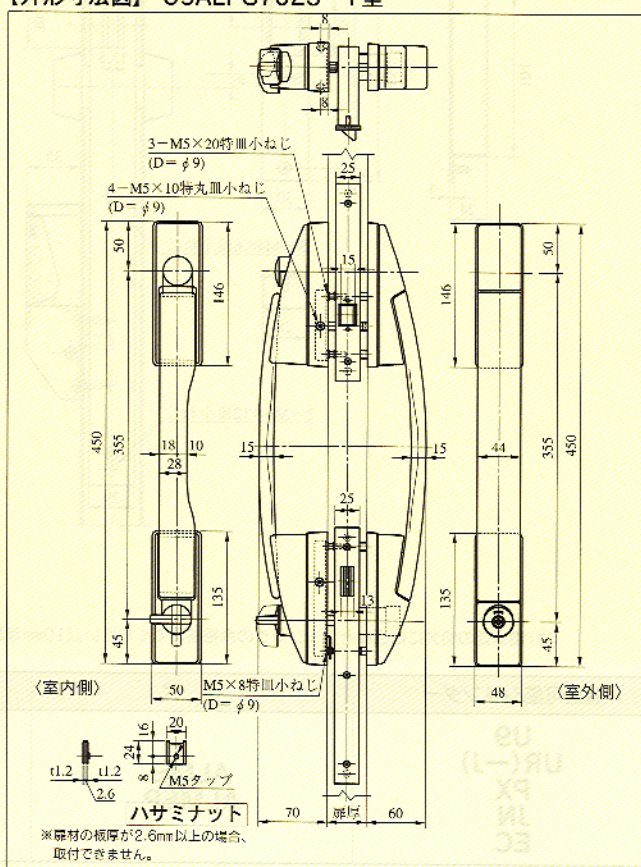
【外形寸法図】 U9ALPG702S-1 型
